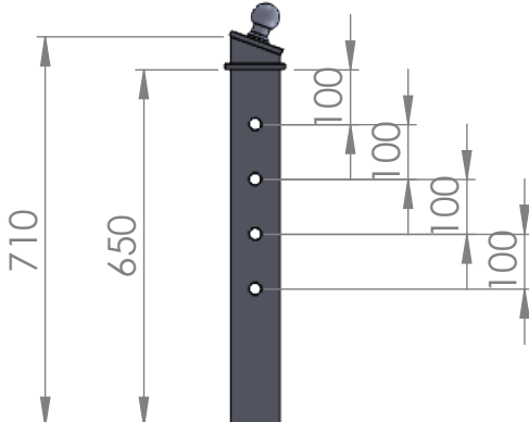
T-12551 - CHANDELLE A ROTULE 90X90 LG650
