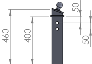
T-12550 - CHANDELLE A ROTULE 90X90 LG400
