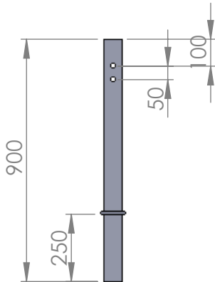
T-12524 - Fourreau 70x70x3 Lg.900 Qté : 4
