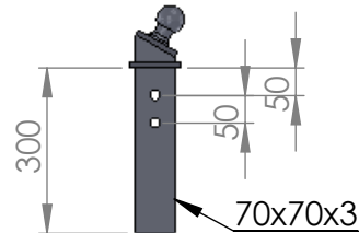
T-12512 - chandelle à rotule 70x70x3 Lg.360 Qté : 2
