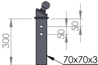
T-12512 - chandelle à rotule 70x70x3 Lg.360 Qté : 4
