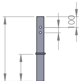
T-12523 - Fourreau 70x70x3 Lg.600 Qté : 4
