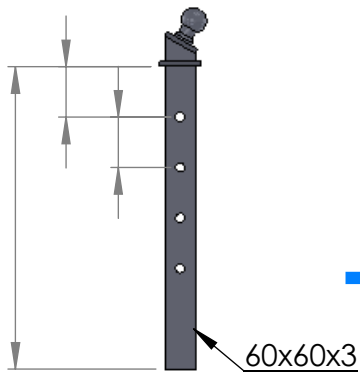
T-12522 - chandelle à rotule 60x60x3 Lg.660 Qté : 4
