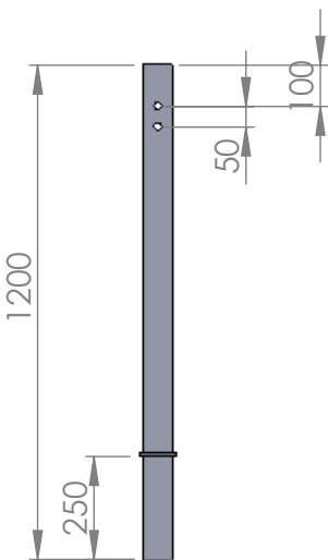
T-12525 - Fourreau 70x70x3 Lg.1200 Qté : 4
