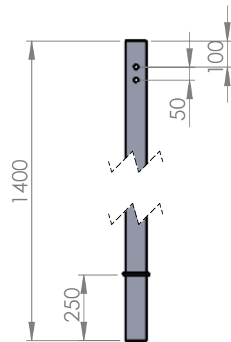
T-12620 - Fourreau 80x80x4 Lg.1400 Qté : 6
