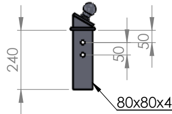
T-12511 - chandelle à rotule 80x80x4 Lg.300 Qté : 6
