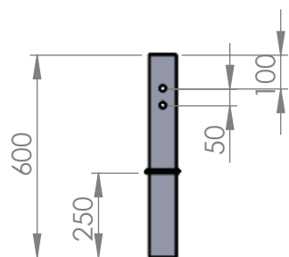
T-12600 - Fourreau 80x80x4 Lg.600 Qté : 6
