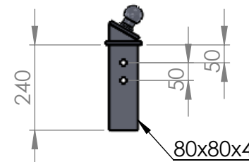
T-12511 - chandelle à rotule 80x80x4 Lg.300 Qté : 4
